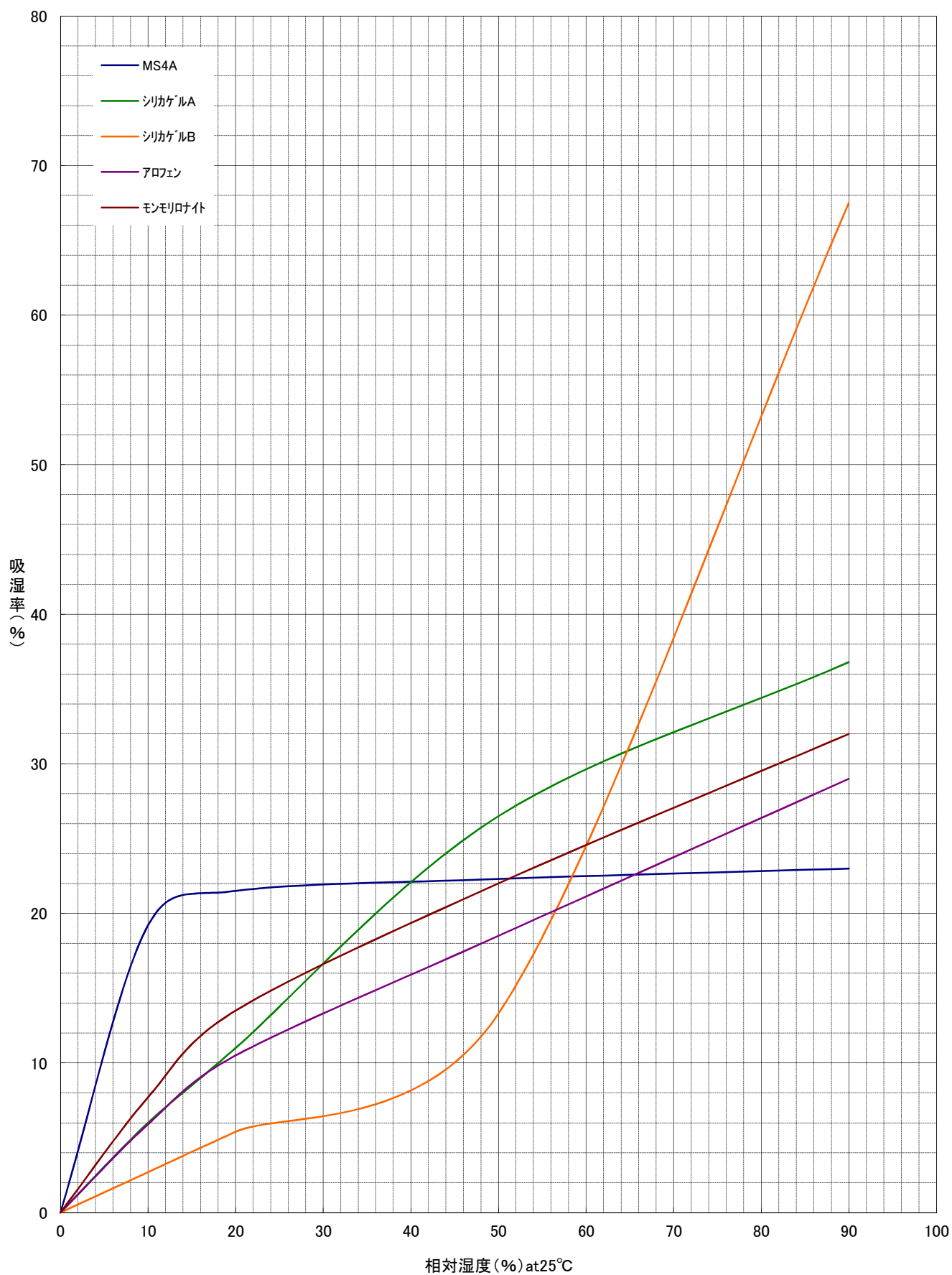
吸湿率比較グラフ
